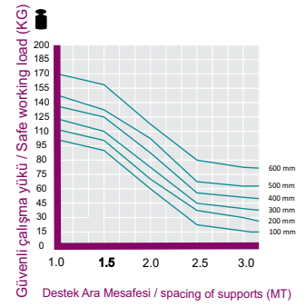
Güvenli çalışma yükü / Safe working load (KG) Destek Ara Mesafesi / spacing of supports (MT)
